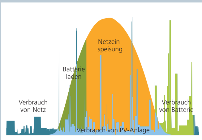
Betrieb Eigenverbrauch: Der Eigenverbrauch wird erhöht (dunkelgrün), das Netz aber nicht entlastet. Quelle: Basler & Hofmann AG
